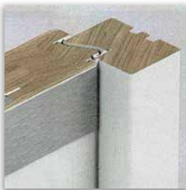
Francouzský rám ze strany závěsů
